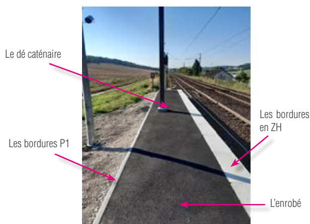
Figure 1 : Allongement de 22,5 m en Voie 2 direction Paris, Gare de Mareil-sur-Mauldre.
